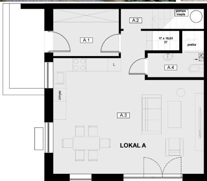
RZUT PARTERU
