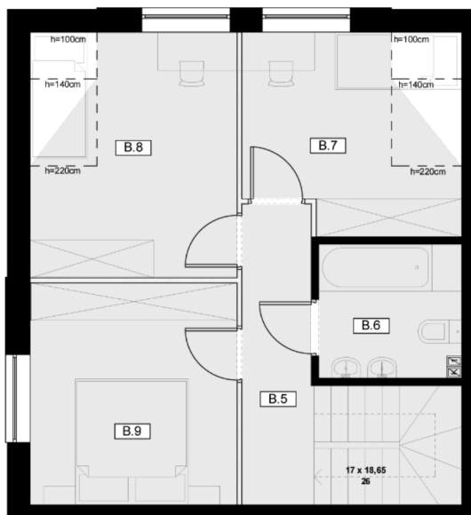
RZUT PIĘTRA
